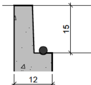
Schemat pokrywy: szczelne połączenie pokrywy ze zbiornikiem
