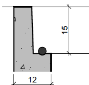
Schemat pokrywy: szczelne połączenie pokrywy ze zbiornikiem
